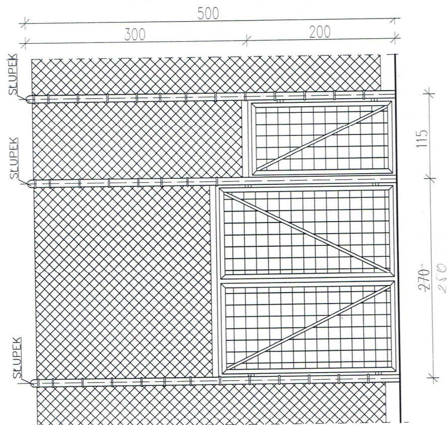
SCHEMAT BRAMY I FURTKI W OGRODZENIU BRAMA 1 szt. FURTKA 1 szt.
